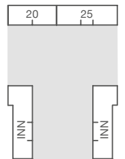
ÉPAISSEUR 250 mm
